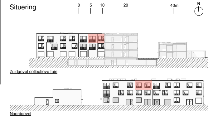
Geveltekeningen
